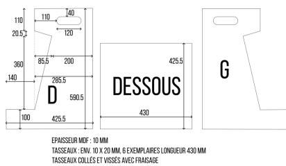
PLAN DE DÉCOUPE DES PIÈCES EN MDF
