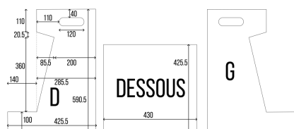
PLAN DE DÉCOUPE DES PIÈCES EN MDF
